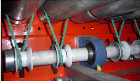
PU Hook belts 88 Sh.A
